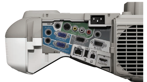
Interfaz EB-470
