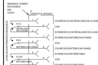
Diagramme de l'interface du contacteur-disjoncteur
